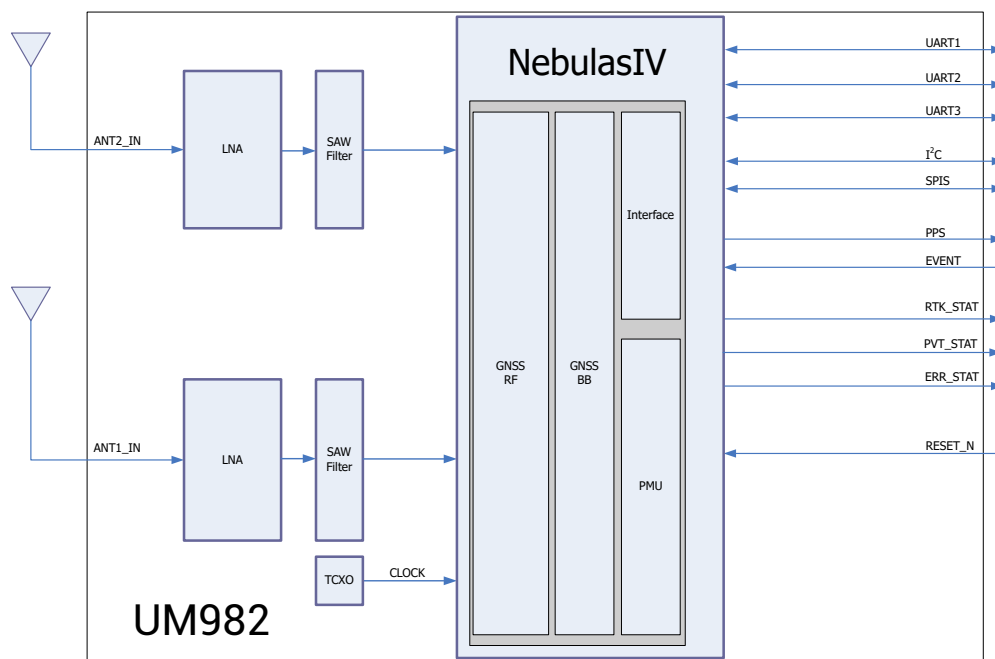
图 1-2 功能框图
