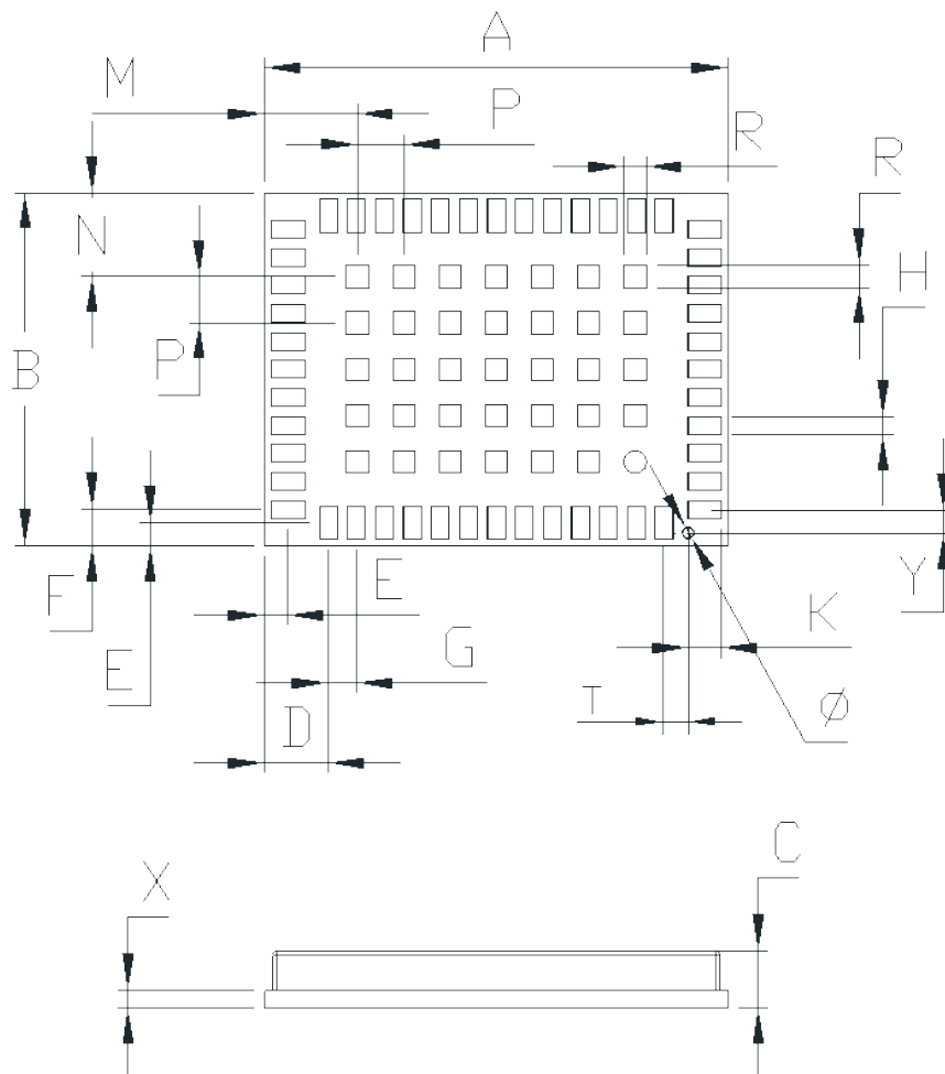
图 2-2 机械尺寸
