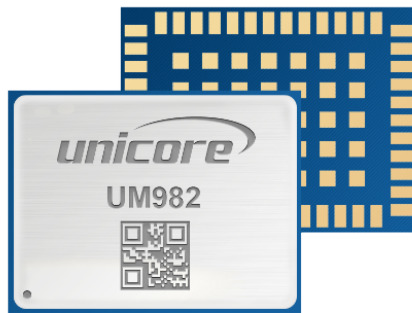
图 1-1 模块示意图
