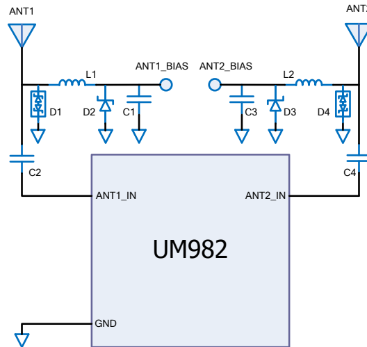
图 3-2 外部天线馈电参考电路图
