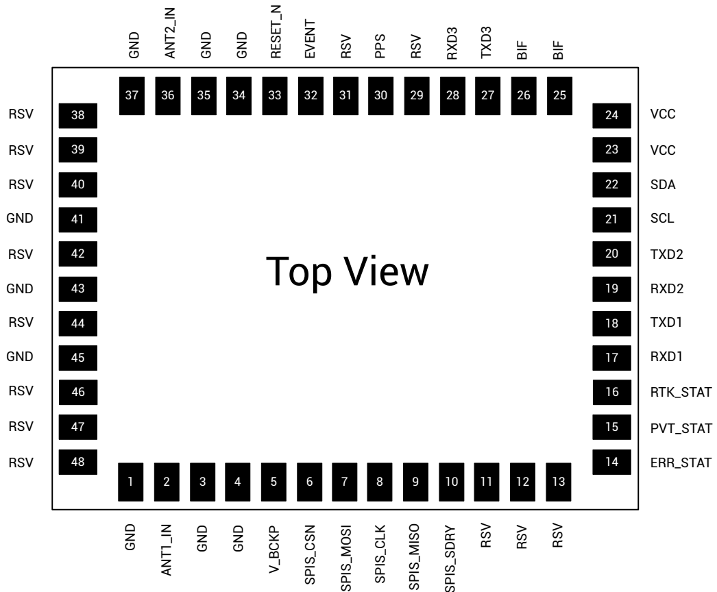
图 2-1 引脚图
