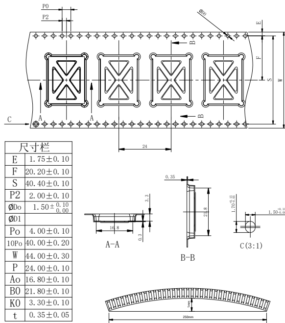
图 5-3 卷装示意图
